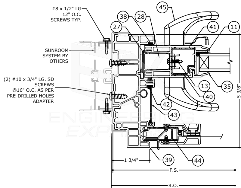
3.3 JAMB DETAIL
