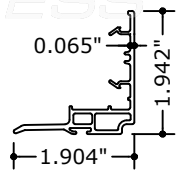
31 7026 INTERLOCK
