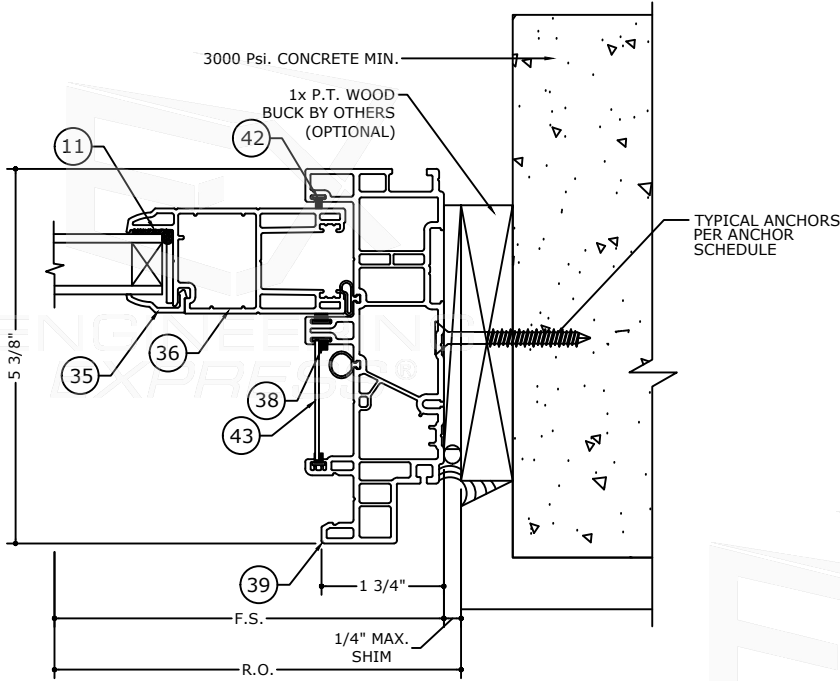
5 JAMB DETAIL SCALE: N.T.S.
