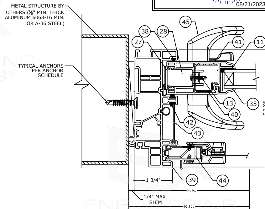
3.2 JAMB DETAIL
