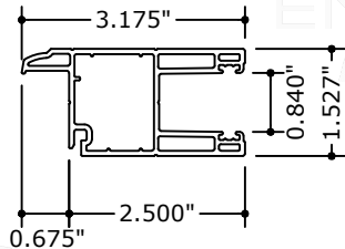
30 7506 CENTER STILE
