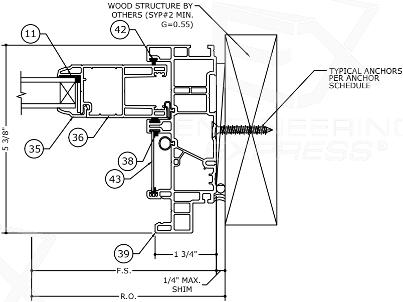
5.1 JAMB DETAIL SCALE: N.T.S.
