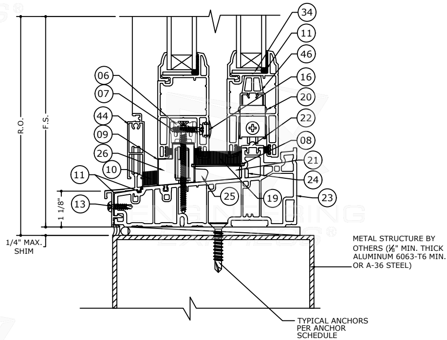
2.2 SILL DETAIL SCALE: N.T.S.
