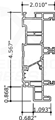
39 7004 JAMB PROFILE
