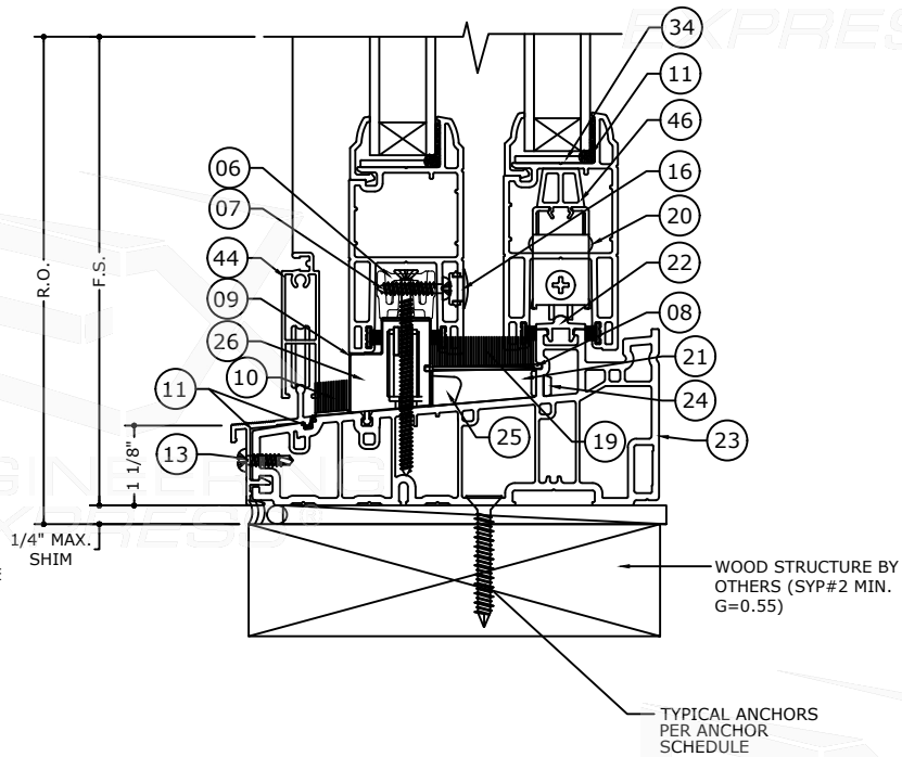
2.1 SILL DETAIL SCALE: N.T.S.
